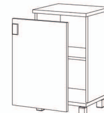
Тумба МР-2431 шир./вис./гл. 0,40/0,67/0,39
