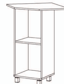
Тумба кутова МР-2426 шир./вис./гл. 0,66/0,92/0,36
