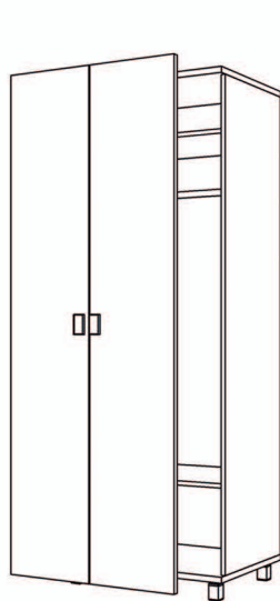
Шафа для одягу Ш-1463 (1467) шир./вис./гл. 0,68/1,93/0,52 (0,36)
