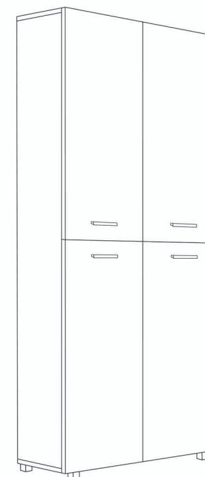
Шафа MP-2897 шир./вис./гл. 0,80/2,045/0,32
