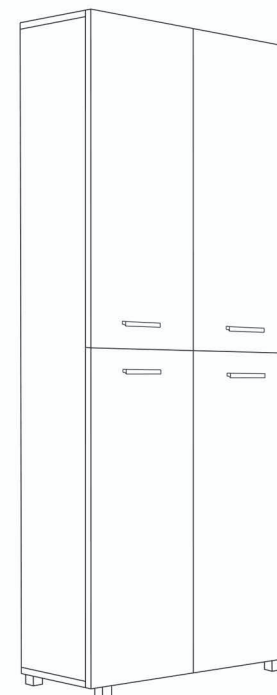
Шафа MP-2898 шир./вис./гл. 0,40/2,045/0,32
