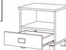
Тумба приліжкова ТБ-293 шир./вис./гл. 0,40/0,43/0,39
