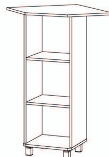
Тумба кутова МР-2413 шир./вис./гл. 0,60/1,08/0,36
