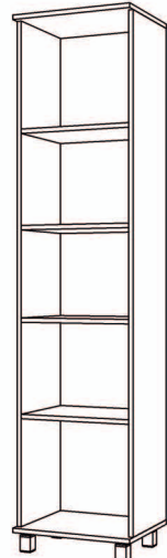
Стелаж СТМ-60 шир./вис./гл. 0,45/1,93/0,36
