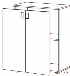
Тумба МР-2433 шир./вис./гл. 0,68/0,92/0,39
