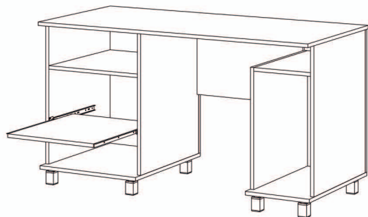
Стіл для комп'ютера СП-498 шир./вис./гл. 1,35/0,76/0,65
