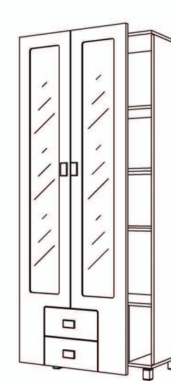
Шафа для книг ШК-326 шир./вис./гл. 0,68/1,93/0,43
